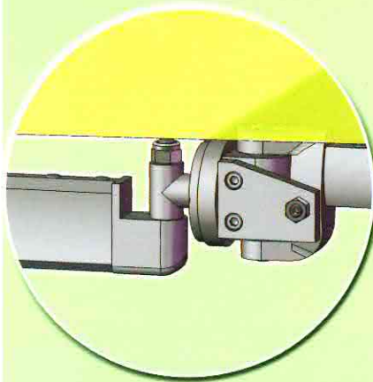
Mehrfach verstellbares Universal-Dreh- und Schwenklager
