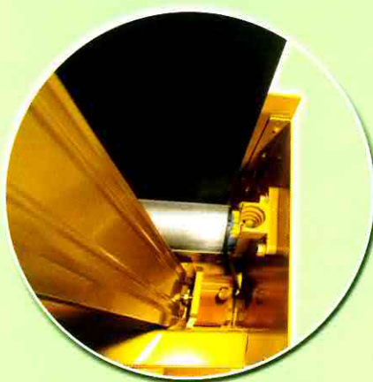
Gelenkiges Excenter-Lager und trichterförmige Führung für passgenaues Schließen der Blende
